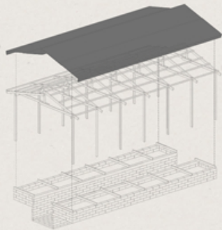
AXONOMÉTRICA DESPEZADA: 1 MÓDULO.
