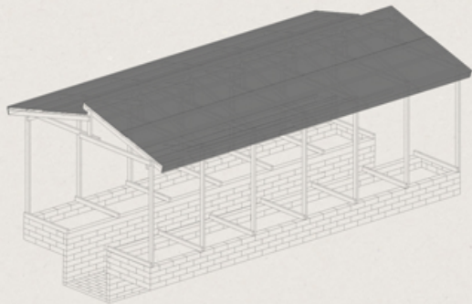
AXONOMÉTRICA: 1 MÓDULO.
